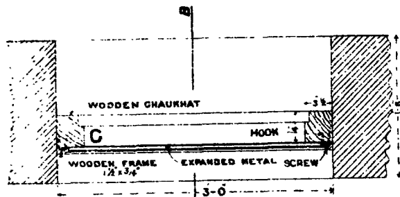
PLAN Fig. 2
