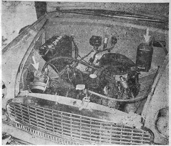
அமெரிக்காவில் பயிற்சி பெற்ற தமிழ் நாட்டுப் பொறியியலர் கண்டுபிடித்த மின் சக்தியால் இயங்கும் 'பியூர் ஸ்டாப்' எனப்படும் மிசேக்கும் (இடதுபுறம் உள்ளது) இயந்திரத்தைக் குவிரவைக்கும் 'நியோகால்' பகுதியும் (வலதுபுறம் உள்ளது) படத்தில் அமைந்திருப்பதை காணலாம்.
